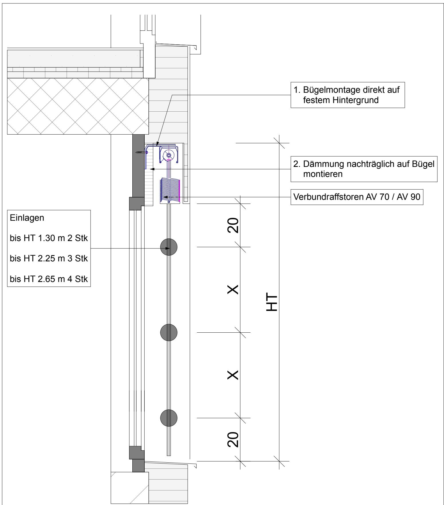
Storendetail Verbundraffstore AV 70 / AV 90
